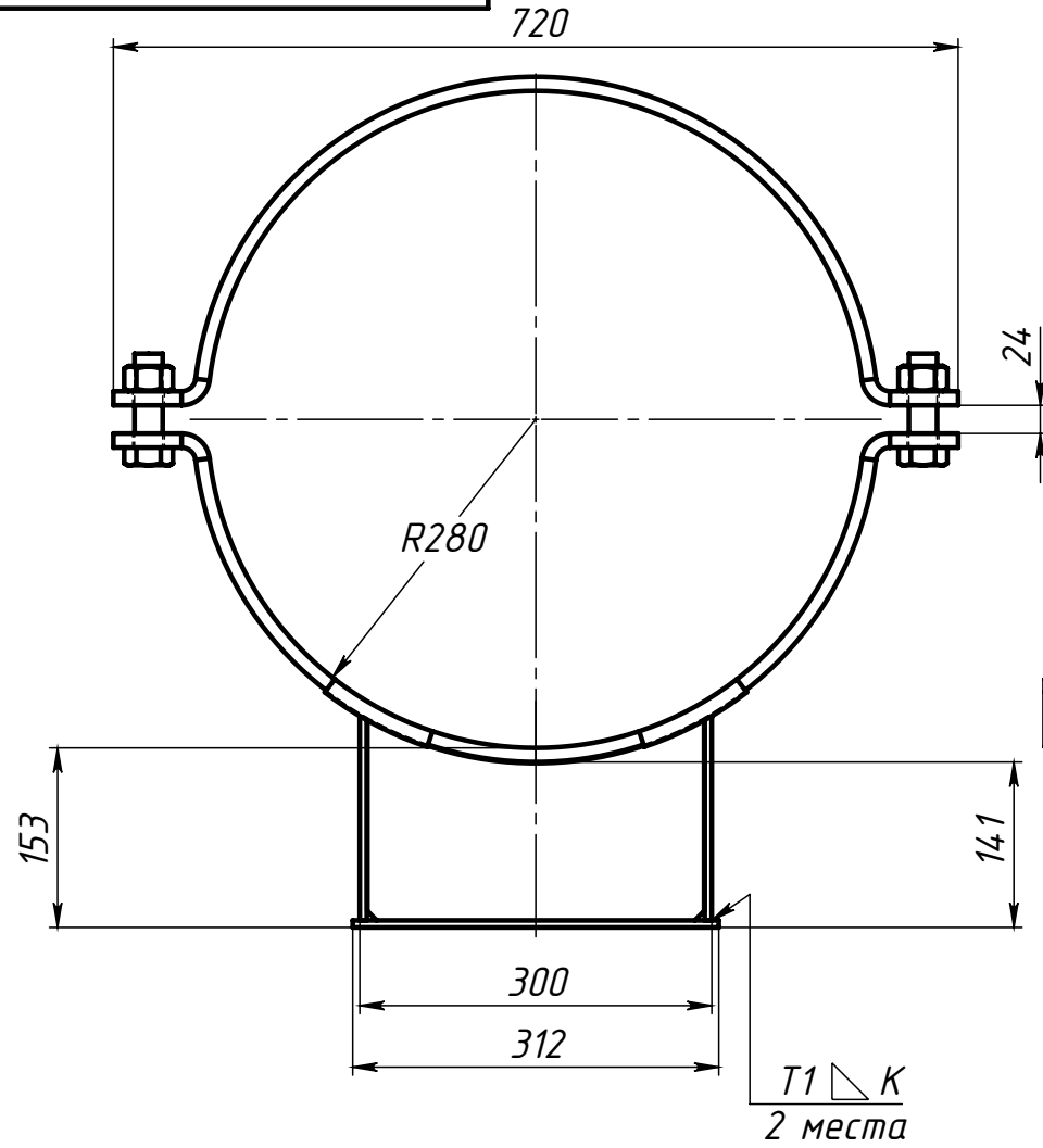
Поз.4 (Полухомут)
