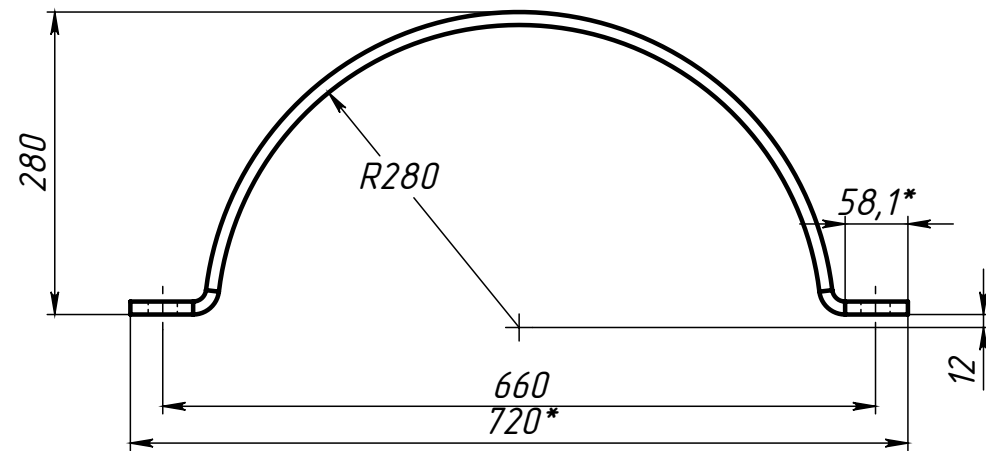
Поз.4 (Полухомут)
